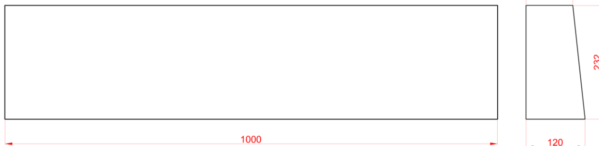
Cordolo TIPO "C"
